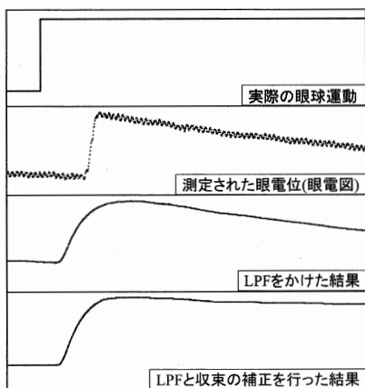
図4: 眼電図とフィルタリングの結果
