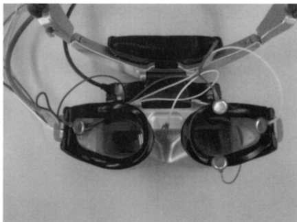
図 2: HMD の接眼部
