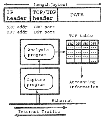
図 1: システム構成図
