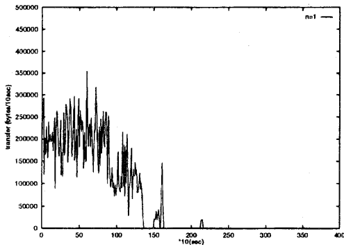
図 3: TCP pair NO.1 のトラフィック
