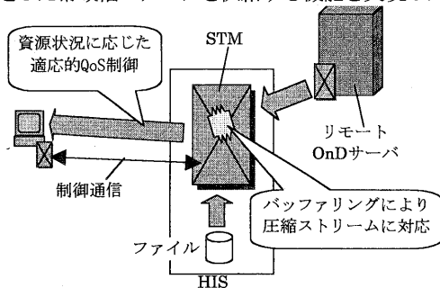
図 7 ストリームバッファリング
