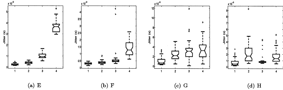
図 8 Jitter for TCP
