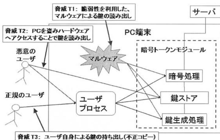
図1. ユーザ認証における脅威
