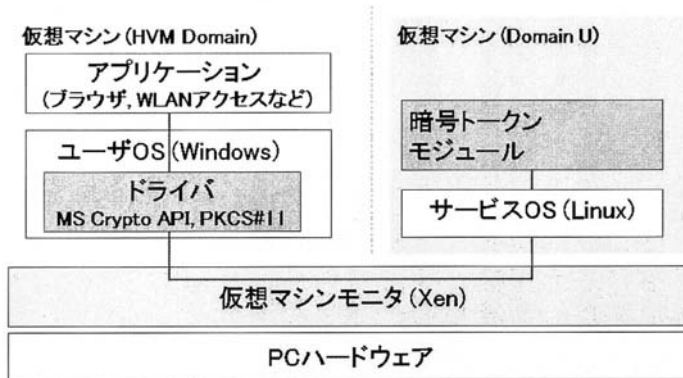
図2. 仮想クレデンシャルコンテナの構成
