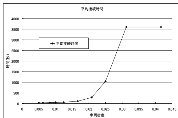
図 10. 接続可能時間
