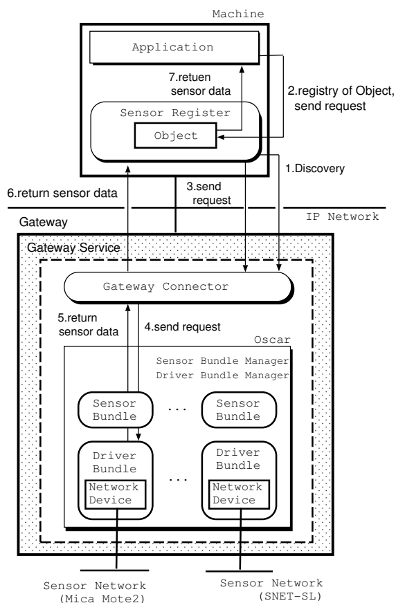
図3 ゲートウェイサービスとアプリケーションの実装
