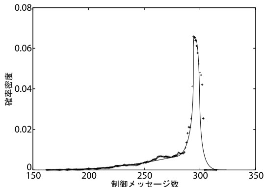
図 8: 制御メッセージ数の分布
