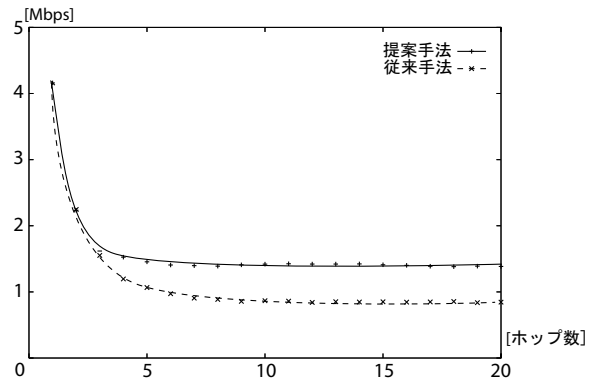
図 7: エンド-エンド帯域幅
