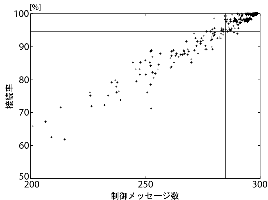
図 9: 制御メッセージ数と接続性
