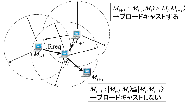
図 6: 経路探索プロトコル
