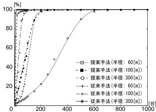
図 10: 経路検出成功率
