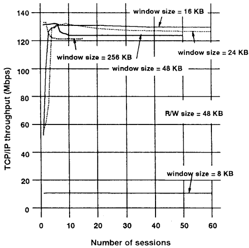
図7 多重送受信性能
