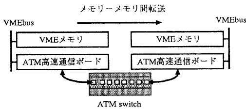
図 5 試験環境
