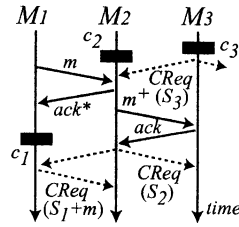
図 5: 誤検出紛失メッセージの多重受理回避 (誤検出でない場合)
