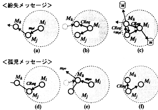
図8: 紛失/孤児メッセージになり得るメッセージ
