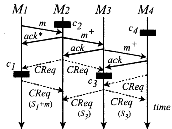
図 7: 紛失メッセージの多重検出の回避
