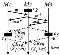
図 4: 誤検出紛失メッセージの多重受理回避 (誤検出の場合)
