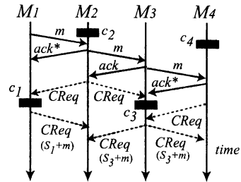
図 6: 紛失メッセージの多重検出
