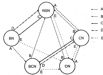
図 3 ノード v_i の状態遷移図
