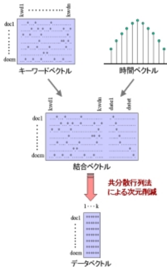
図 1: ベクトル作成手順
