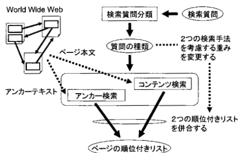
図 1: Web 検索システムの概要
