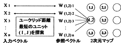
図3：最近ユニットの探索
