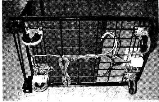
図9 カートの底面。後輪 (左) の回転を測定する。また先頭部分 (右) にはRFIDリーダが取り付けられ、床の上のRFIDタグを読みとる。
