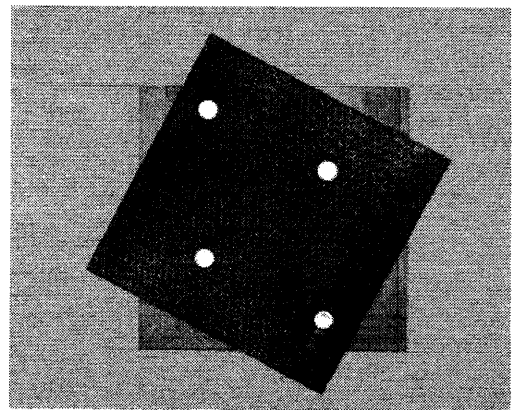
図3. RFIDを裏に取りつけたIDカーペット。1枚のタイルカーペットに4個のRFIDタグを取りつけた。
