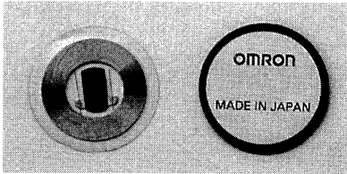
図1. 本研究で使用したRFIDタグ(右)とその内部(左)。直径23mm, 厚さ1.2mmの円盤型。
