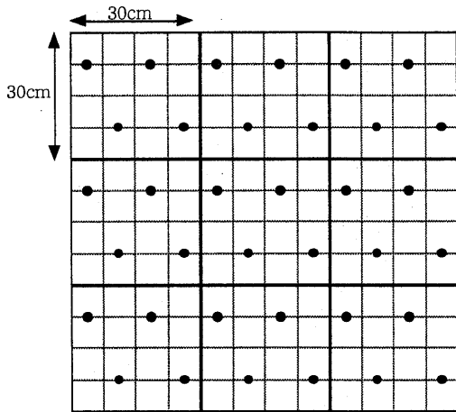
図4. カーペットに取りつけたRFIDタグ(黒丸)の配置。RFIDタグの干渉を減らす効果と、廊下など人が直進する場所での検出率を向上させる効果を得らって、RFIDタグを交互に配置した。
