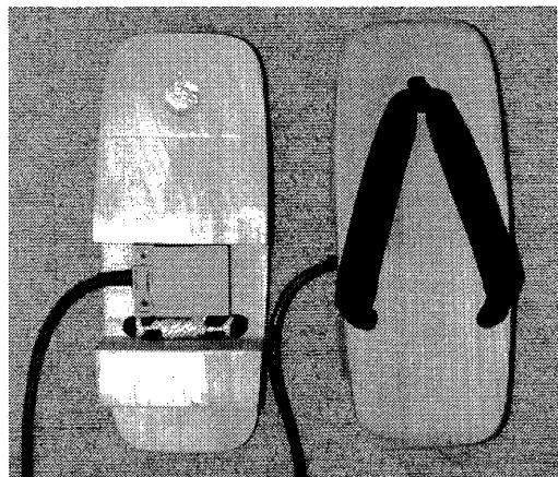
図5. RFIDリーダを取りつけた履き物。床のRFIDタグを読み取ることでユーザの位置を検出する。
