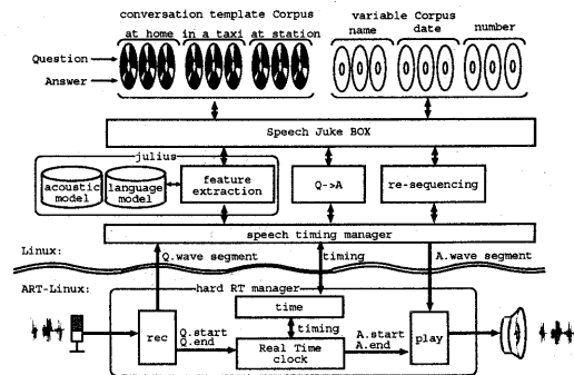
図1: システム構成イメージ
