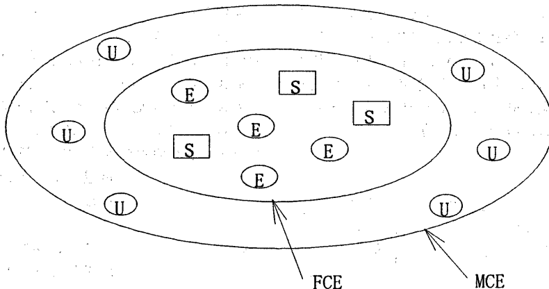
図. 5 MCEモデル
