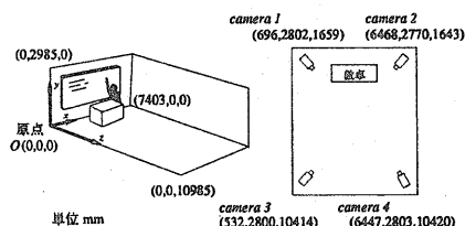
図2: 対象空間とカメラの配置 (単位 mm)
