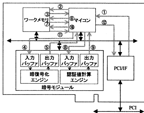
図5 データフロー (IP パケット→IPsec パケットの場合)
