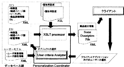
図 9：データフロー図
