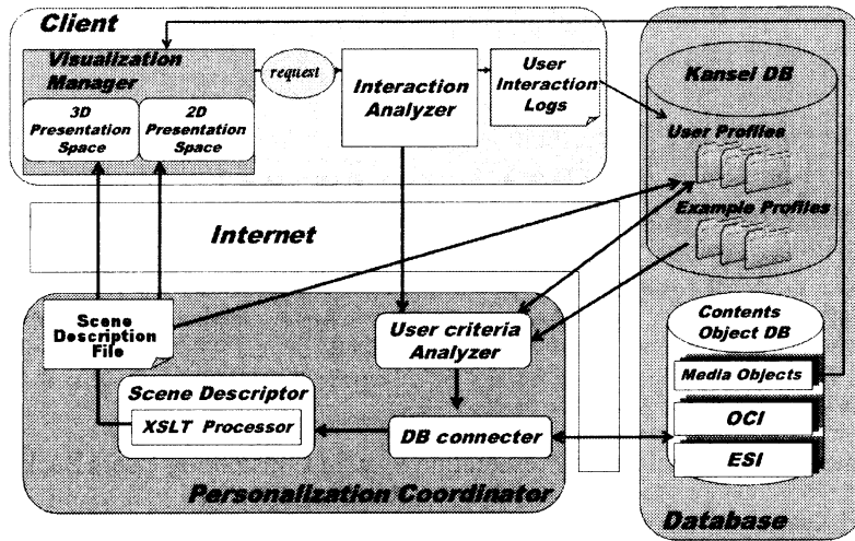
図 1:システムアーキテクチャ
