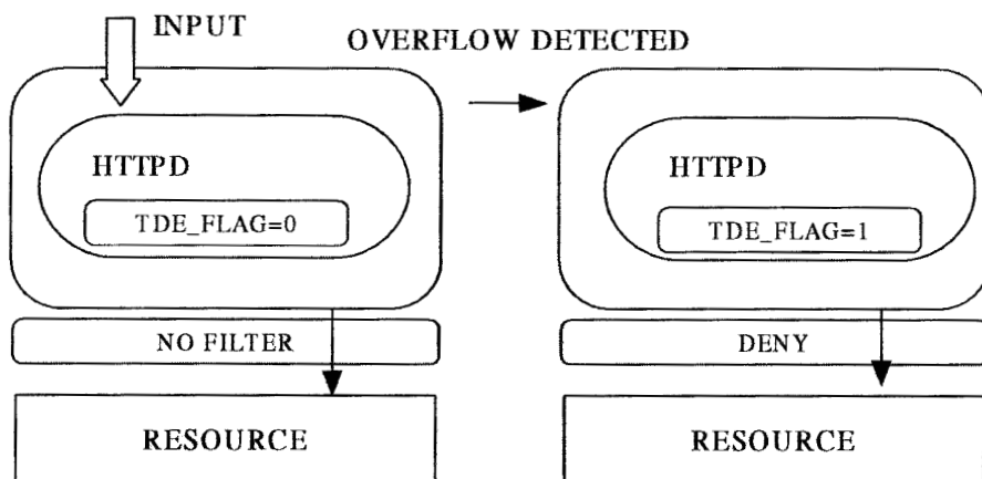
図 2: (悪意のある入力により) オーバーフローが起きたときに、拡張したプロセス構造体の TDE のフラグを立てて、リソースのアクセス禁止を明示的に設定する。
