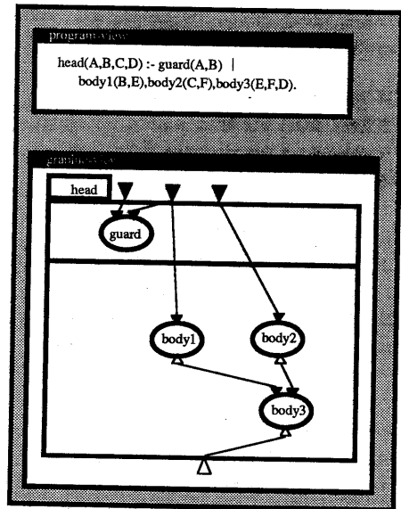
図1 PB '92の画面イメージ
