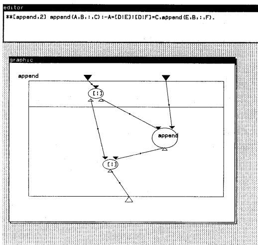
図4 FE '92 によるappendプログラムの入力例
