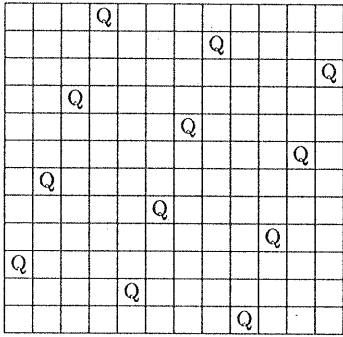
図 8: Yaglom の解の拡張 ( Y_{12}^3 )
