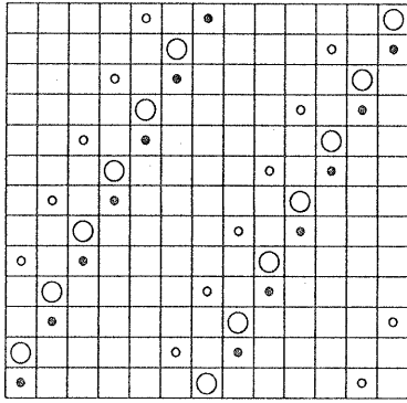
図 5: 基本解の平行移動 ( N = 13 )
