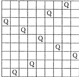
図 16: Falkowski らの N \equiv 9 \pmod{24} の場合の解 ( N = 9 )
