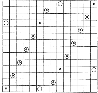
図 9: 基本解への駒の追加と行の交換 ( N = 14 )
