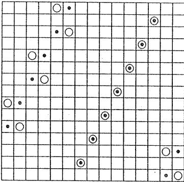
図 19: 行の交換と平行移動による解 ( N = 15 )
