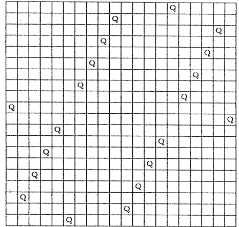
図 10: Yaglom の解の拡張 ( Y_{20}^{10} )
