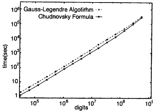
図 4: Chudnovsky の公式と Gauss-Legendre の公式の比較
