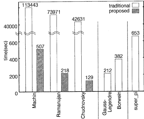
図3: 104万桁の \pi の計算時間
