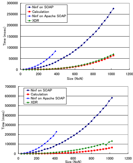
図 4 Ninj on SOAP の性能 (上段: LAN, 下段: WAN)
