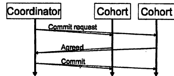
図2 2相コミットのメッセージダイアグラム
