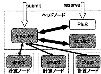
図 4 GridEngine 向け PluS の構造
