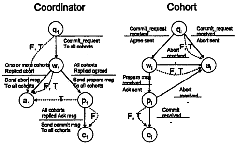
図 5 3相コミットプロトコル
