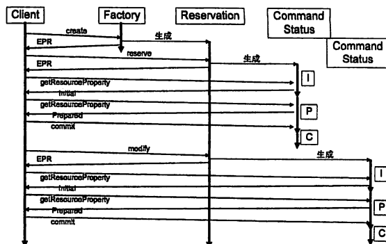
図3 予約インターフェイスのメッセージダイアグラム
