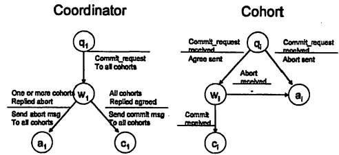
図1 2相コミットプロトコル
