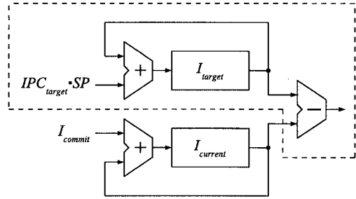
図 2 スループット比較回路
