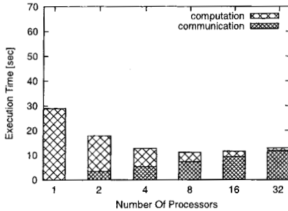
図7 MPIによる4000x4000の行列積実行時間
