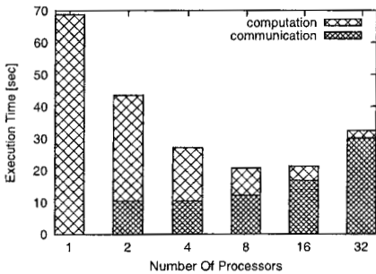
図8 MatlabMPIによる4000x4000の行列積実行時間
