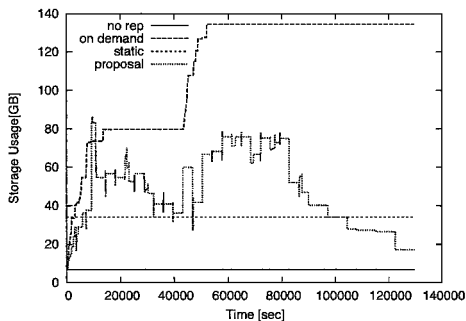
図4 ストレージの使用量の変化
