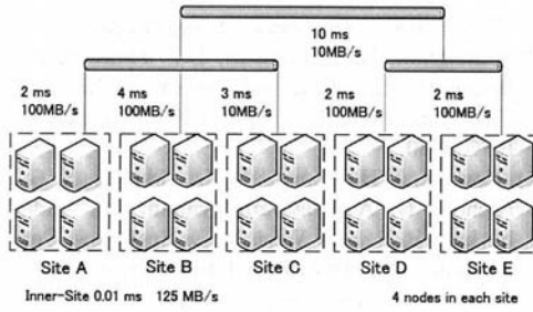
図1 シミュレーションの構成
