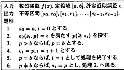
図2 定義域の不等区間への分割アルゴリズム
