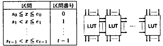
(a) 区間指定関数
