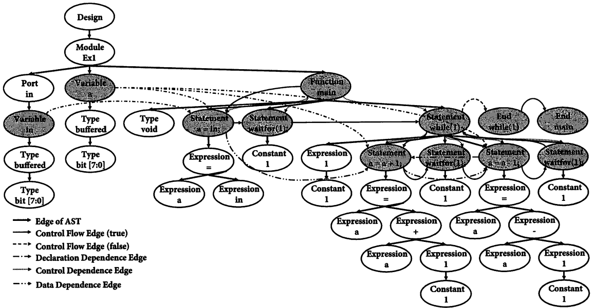
図2 拡張システム依存グラフ ExSDG の例 [10]
