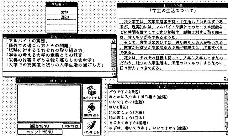
図7 文章化
