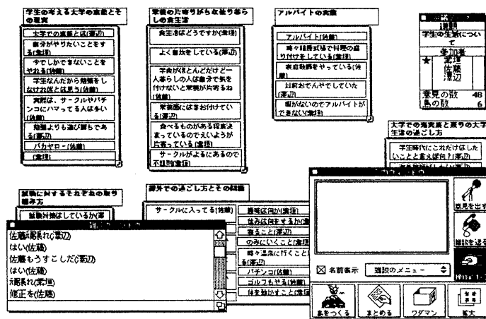
図6 島作成
