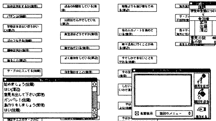
図5 意見入力
