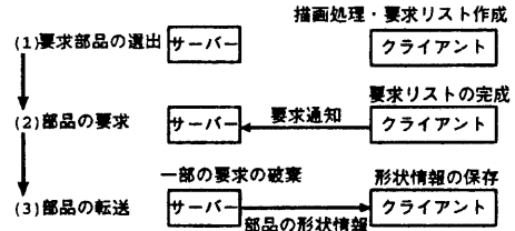
図 2: 要求伝送方式
