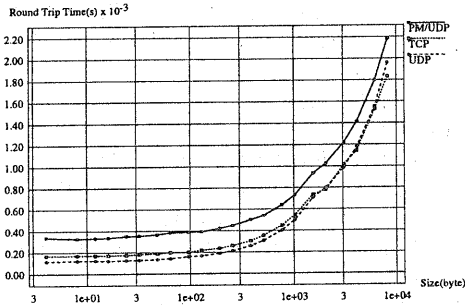
図3 PM/UDPのラウンドトリップ時間
