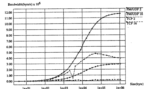
図6 MPI: Allgather
