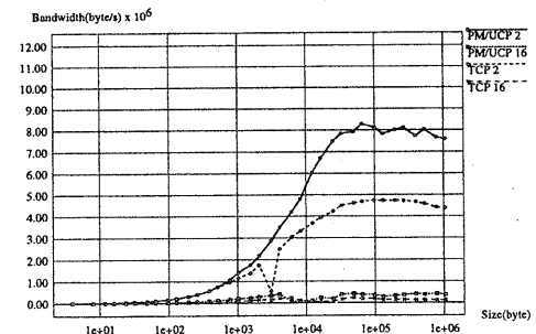
図7 MPI: Alltoall
