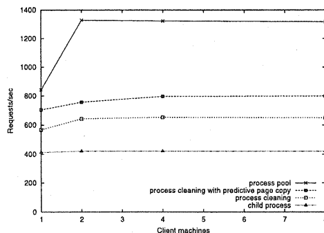
図 3: サーバのスループットの変化
