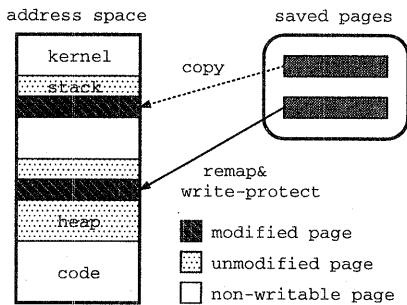
図 1: メモリ状態の復元
