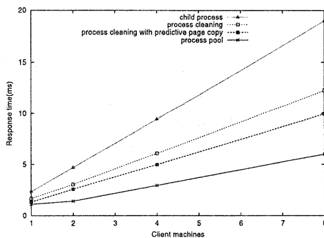
図 2: サーバの平均応答時間の変化
