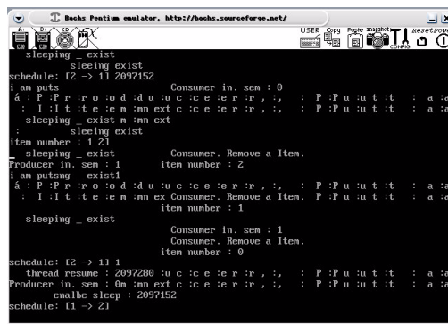
Bochsの画面
