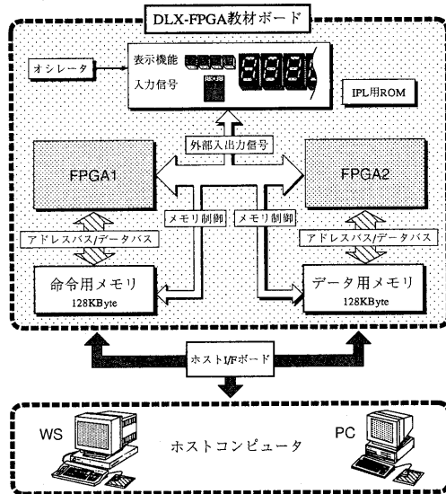
図 3: DLX-FPGA 整数パイプライン実装環境
