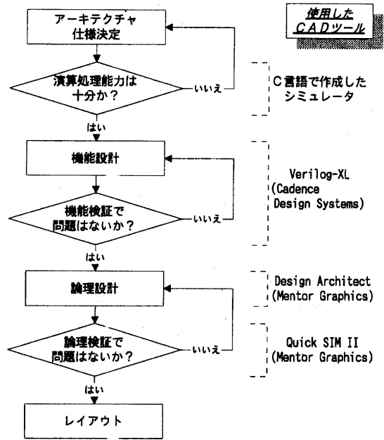
図-3 設計フローとCADツール
