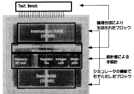
図-6 論理検証モデル
