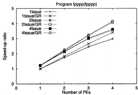
図 4: FPPPP における速度向上率
