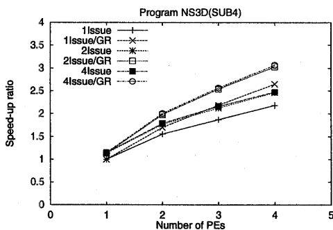
図 3: NS3D における速度向上率
