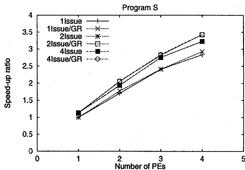
図 2: ランダムスパースマトリクスにおける速度向上率
