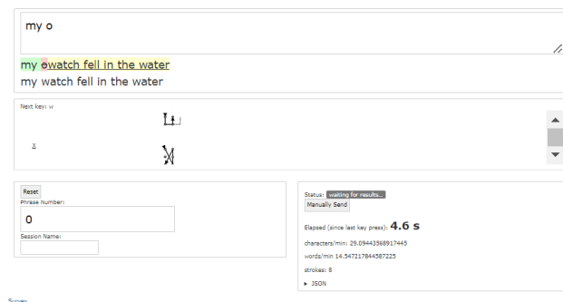
図 6 ユーザテスト用ウェブアプリケーション。
