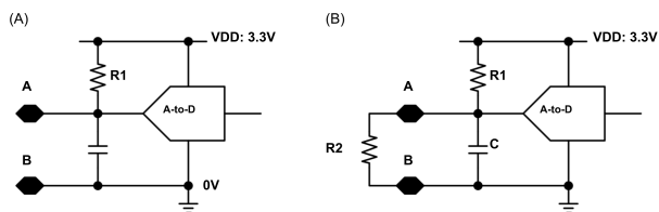
図 3 回路構成。(A) 指が触れていないとき (B) 触れているときの抵抗式タッチセンサの回路モデル。
