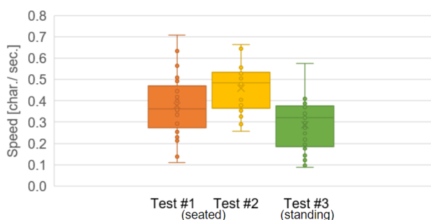
図 7 Yarnkey の入力速度 ( n = 5 )。エラーバーは最大値と最小値 (外れ値は除く)。箱の上下は 75%および 25%パーセンタイル。
