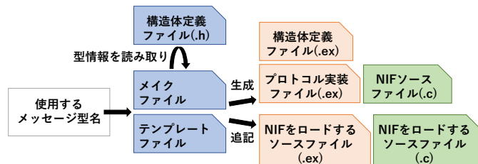
図 4 ソースファイル自動生成フロー
