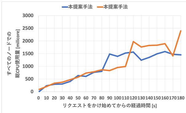
図 12 試行回数を 1000 回にした際の総 CPU 使用量の推移
