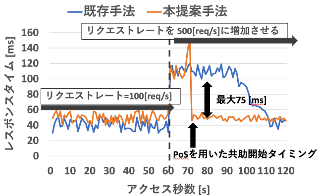
図 13 PoS システムを用いたときのレスポンスタイムの維持
