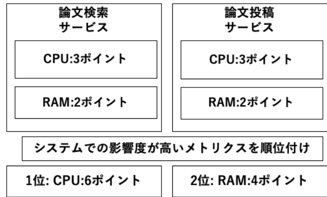
図3 アプリケーション全体でメトリクスの順位付け
