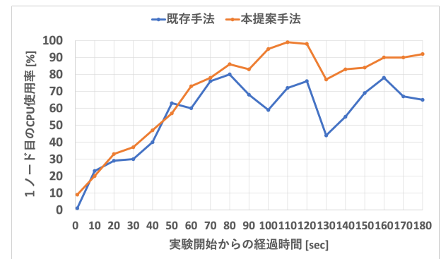
図 11 試行回数を 1000 回にした際の 1 つ目のノードの CPU 使用率の推移
