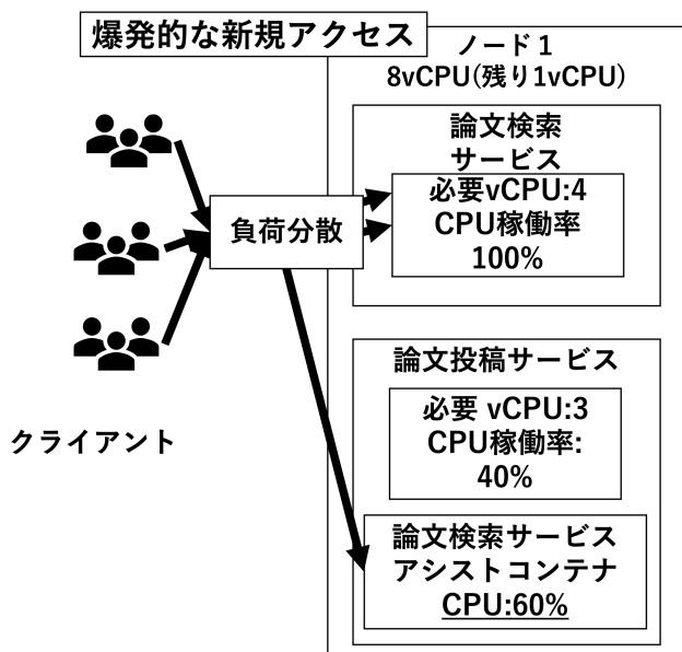
図 5 同一ノード内の使用していない CPU を用いることでノードの CPU 使用率を向上させる。
