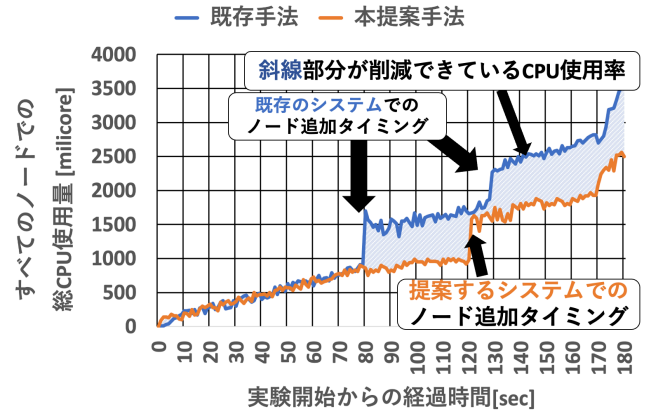
図 10 すべてのノードにおける CPU 総使用量
