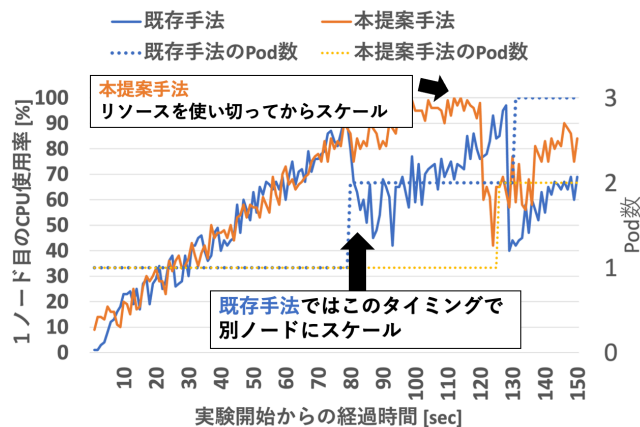
図 9 2 手法での 1 ノード目で計測した CPU 使用率
