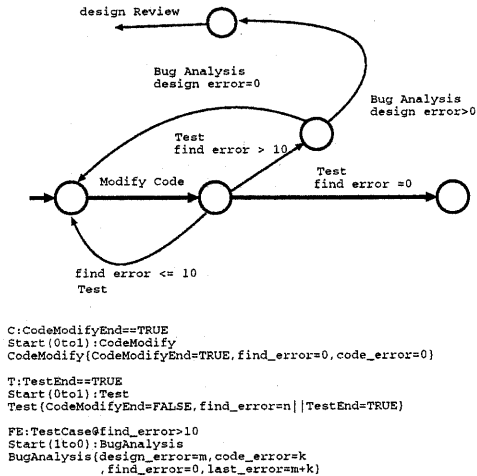
図 9: フィルタの例 (コード修正, テスト)
