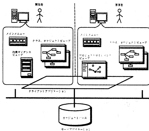
図 13: システム概要図
