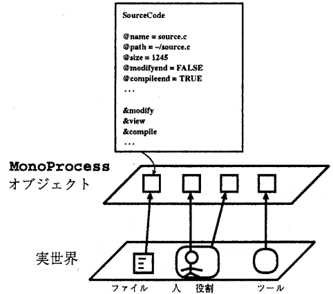
図 1: プロセスモデル MonoProcess の概要図
