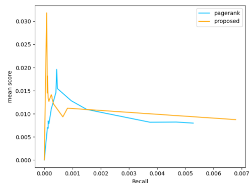
図 5: PageRank 及び提案手法における Recall と平均 escore の関係
