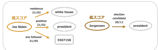
図 3: クエリベクトル設計のための基本アイデア. より直近に, 多くの編集が行われたエンティティに高い値を与える.
