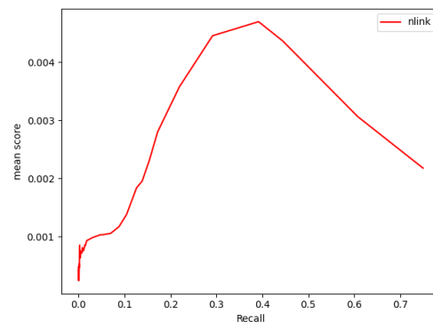
図 4: リンク数を用いる手法における Recall と平均 escore の関係
