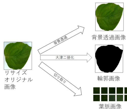
図4 背景透過画像, 輪郭画像, 葉脈画像の作成手法
