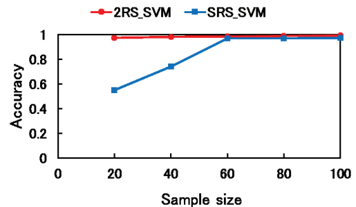
図 10 SRS と 2RS による SVM の正解率 ( D = 2 )
