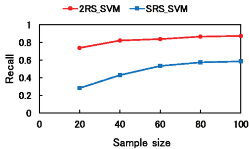
図 11 SRS と 2RS による SVM の再現率 ( D = 4 )
