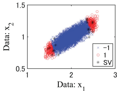
図 8 2RS で学習した SVM によるラベルの推定値
