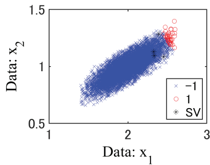
図 7 SRS で学習した SVM によるラベルの推定値
