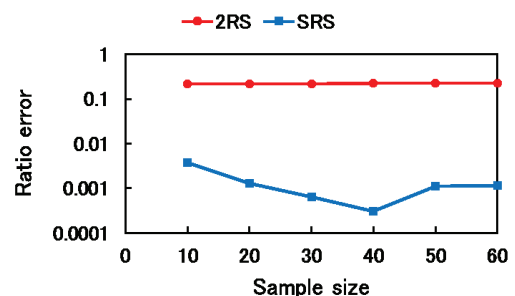
図6 教師データによる母比率の推定誤差
