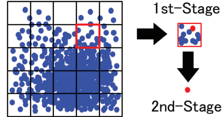
図 2 2 段階無作為抽出法による標本の選択
