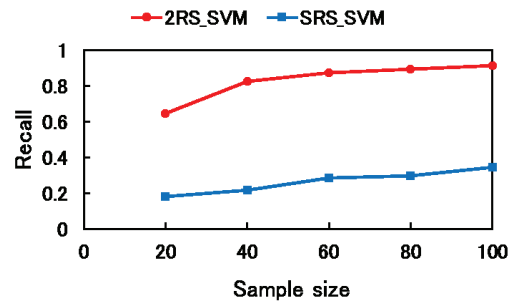
図 9 SRS と 2RS による SVM の再現率 ( D = 2 )
