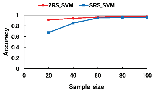
図 12 SRS と 2RS による SVM の正解率 ( D = 4 )
