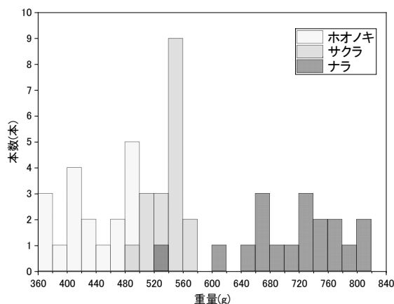
図 4 測定結果
