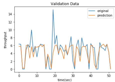
図 12 テストデータによる予測 (端末 1)
