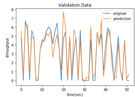
図 14 テストデータによる予測 (端末 3)
