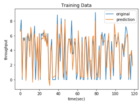
図 9 学習データによる予測 (端末 3)
