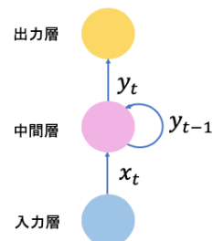
図 4 RNN のモデル
