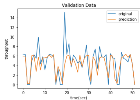
図 13 テストデータによる予測 (端末 2)
