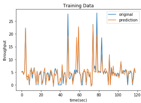
図 11 学習データによる予測 (端末 5)
