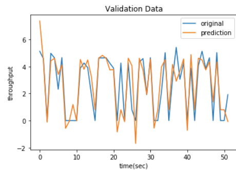
図 15 テストデータによる予測 (端末 4)
