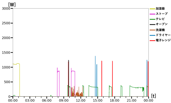
図 2: 家電ごとの個別の消費電力
