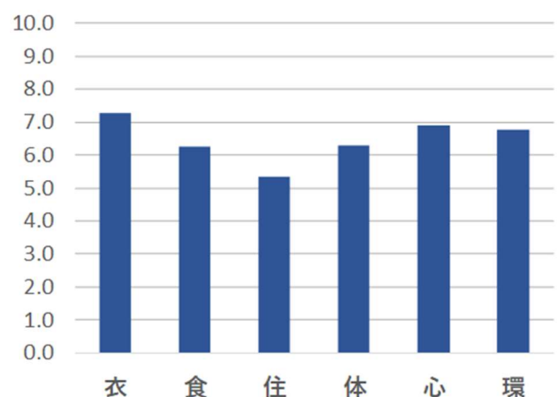
図6 全体の平均
